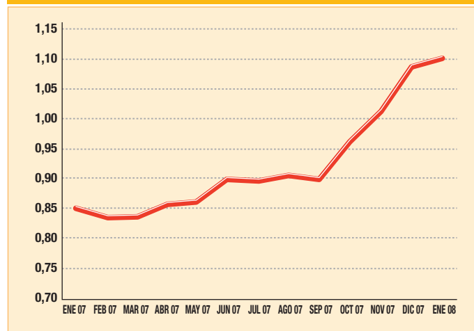
GRAFICO 2. EVOLUCIÓN DEL PRECIO DEL PROPANO (EUROS/KG)
